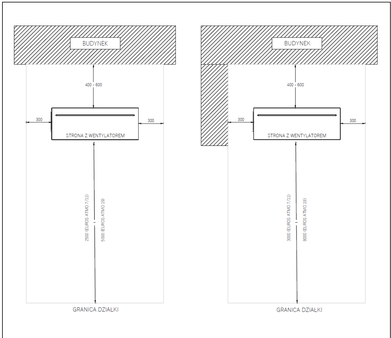
Rys. 9: Ograniczenia dotyczące miejsca ustawienia jednostki zewnętrznej pompy ciepła EUROS ATMO (wymiary w mm).
