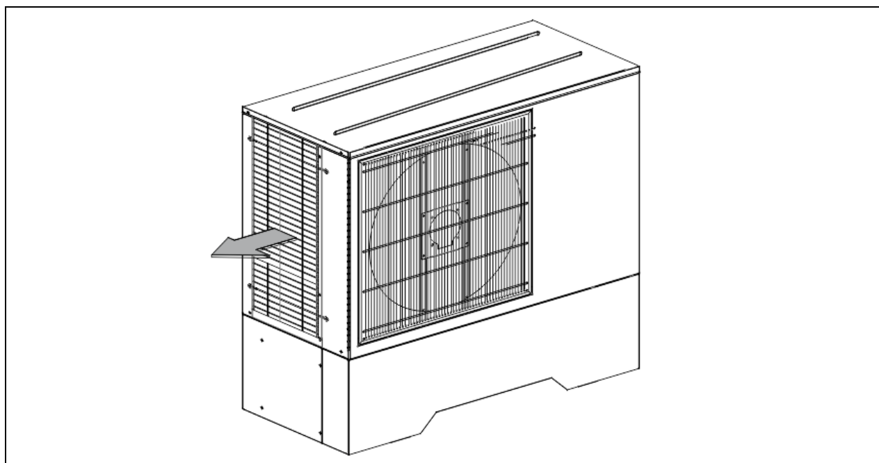
Rys. 12: Sposób zdjecia kratki zabezpieczajcej w jednostce zewnętrznej pompy ciepła EUROS ATMO.
