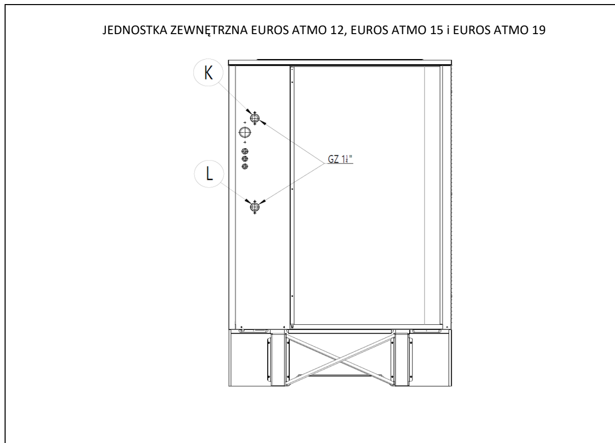
Rys. 11: Przyłącza hydrauliczne jednostki zewnętrznej pompy ciepła EUROS ATMO 12, EUROS ATMO 15 i EUROS ATMO 19.
